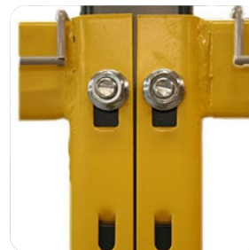
UNARCO T-Bolt
